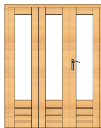
DL01H 1495 x 1935 (vouw)
