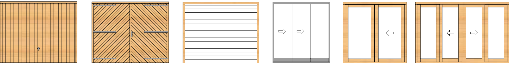
GD01 2290 x 2000 (kantel) Keteldruk geïmpregneerd (bruin) GD02 2290 x 2000 (openslaand) GD03 2290 x 2000 (sectionaal) Glasschuifwand in elke breedtemaat leverbaar SD200 2000 x 1935 (schuif) SD300 3000 x 1935 (schuif)
