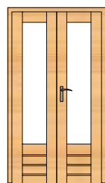
PE26 1000 x 1800 PE26H 1000 x 1935
