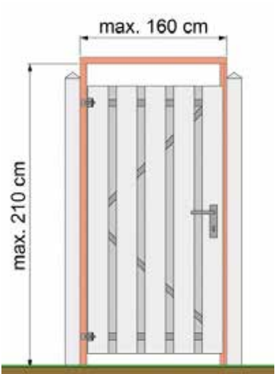
Douglas tuindeurkozijn max. 160x210 cm 29798
