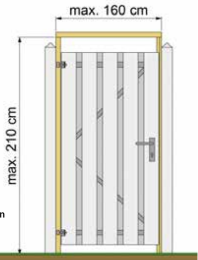
Naaldhout Tuindeurkozijn max. 160x210 cm 29573
