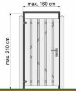
Naaldhout tuindeurkozijn zwart geïmpregneerd max. 160x210 cm 29815
