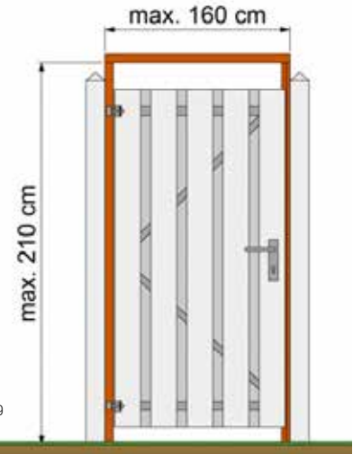
Hardhouten tuindeurkozijn max. 160x210 cm 29799
